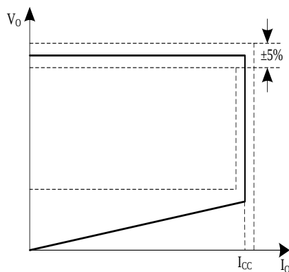
CC/CV 曲线
