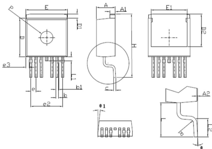
TO263-7
