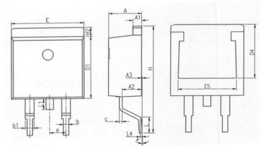
TO-263 Package
